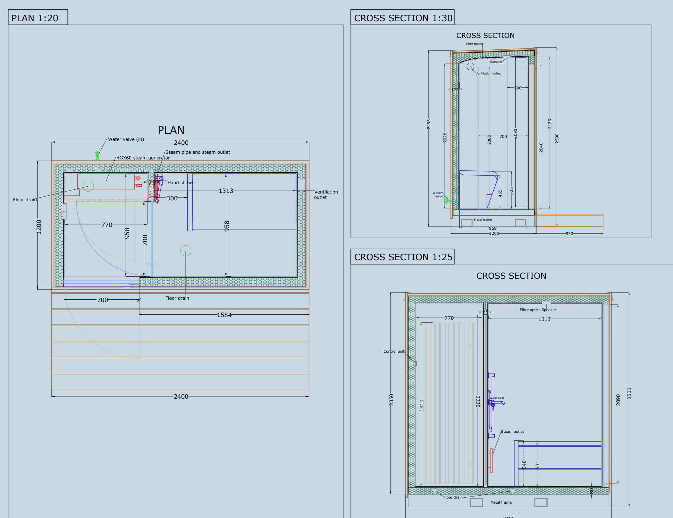
KUUT STANDARD steam room 1,2x2,4
